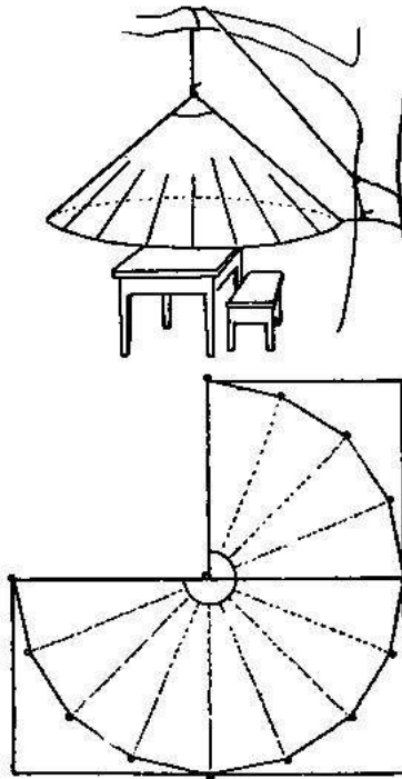
Fig. 11. Sibley awning
